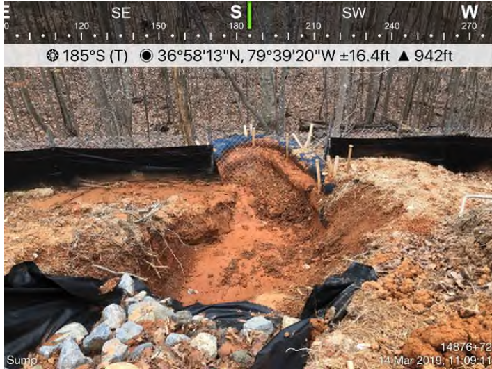
Fig. 11: STA 14876+72 – Maintain/cleanout sump.
